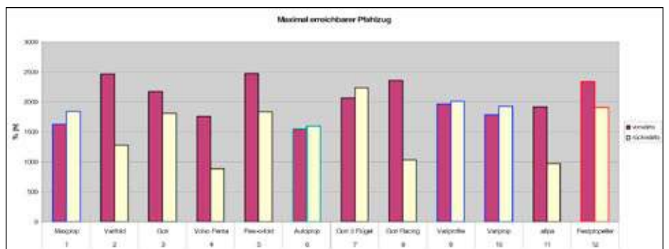
Die Pfahlzugwerte ändern sich teilweise sehr: zwei Props sind an der 2500N-Marke
