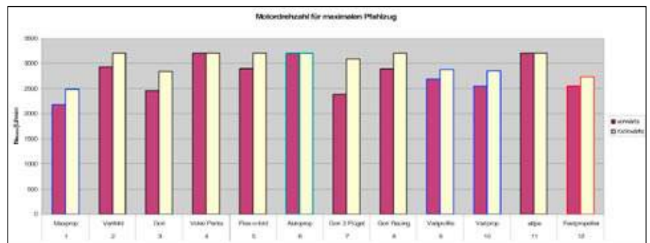
Jetzt liegt die erforderliche Drehzahl für die maximalen Pfahlzugwerte höher als zuvor
