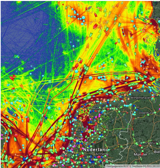
Figuur; SOTDMA cellen
