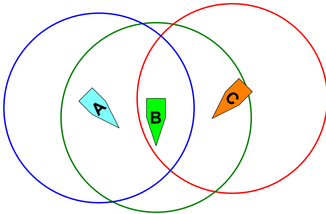
Figuur; SOTDMA cellen
