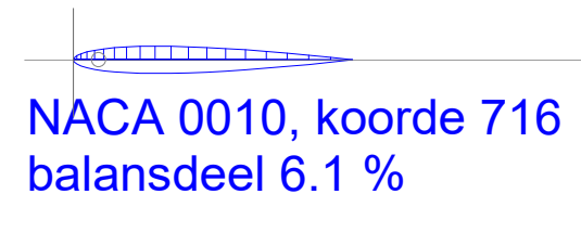
Zelfde maar minder breed oppervlakte 1,08 m 2 roerverhouding 2,46
