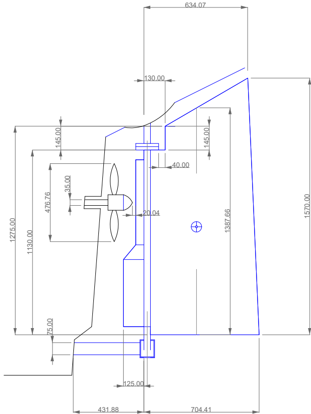
Origineel oppervlakte 1,00 m 2 roerverhouding 1,93
