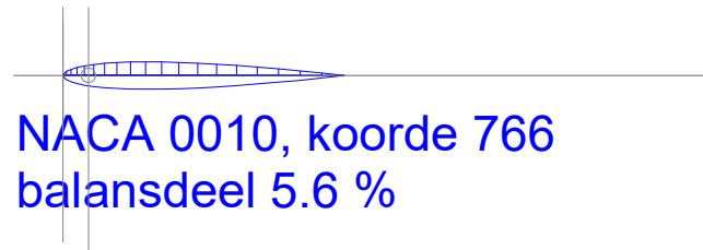
Met gewijzigde hoogte oppervlakte 1,17 m 2 roerverhouding 2,30
