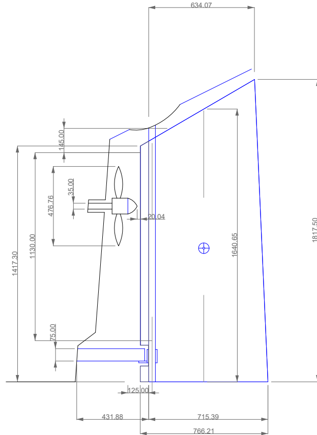
Met gewijzigde hoogte oppervlakte 1,17 m 2 roerverhouding 2,30
