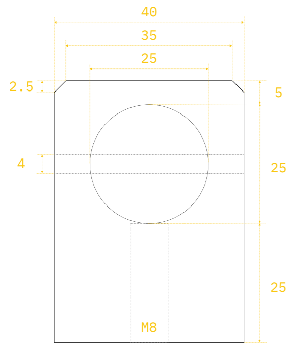
Vooraanzicht
