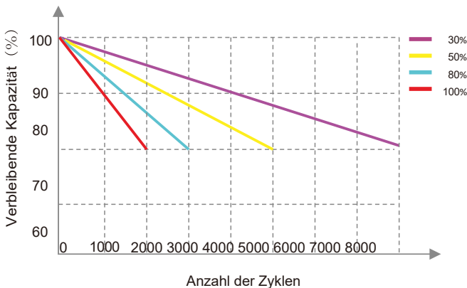
DoD-Entladezyklen(1C)
