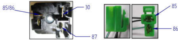
Detalle relé bujías precalentamiento / Preheating relay
