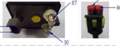
Detalle relé de aislamiento / Isolating relay
