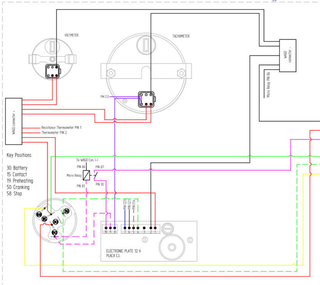
Detalle relés de arranque / Starter relay
