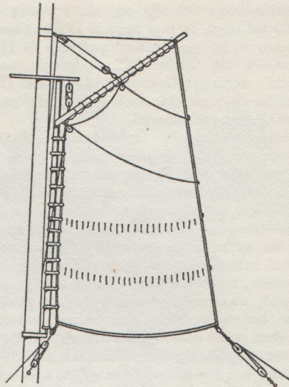
De geitouwen waarmee het achterlijk van de bezaan tegen de gaffel wordt opgehaald (n. Le Comte, Praktikale zeevaartkunde, 1842)
