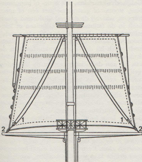
De geitouwen (1) aan de achterzijde van een marszeil, waarmee de schoothoorns (2) worden opgehaald
